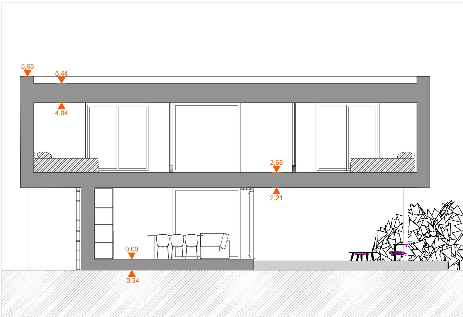
Coupe BB
