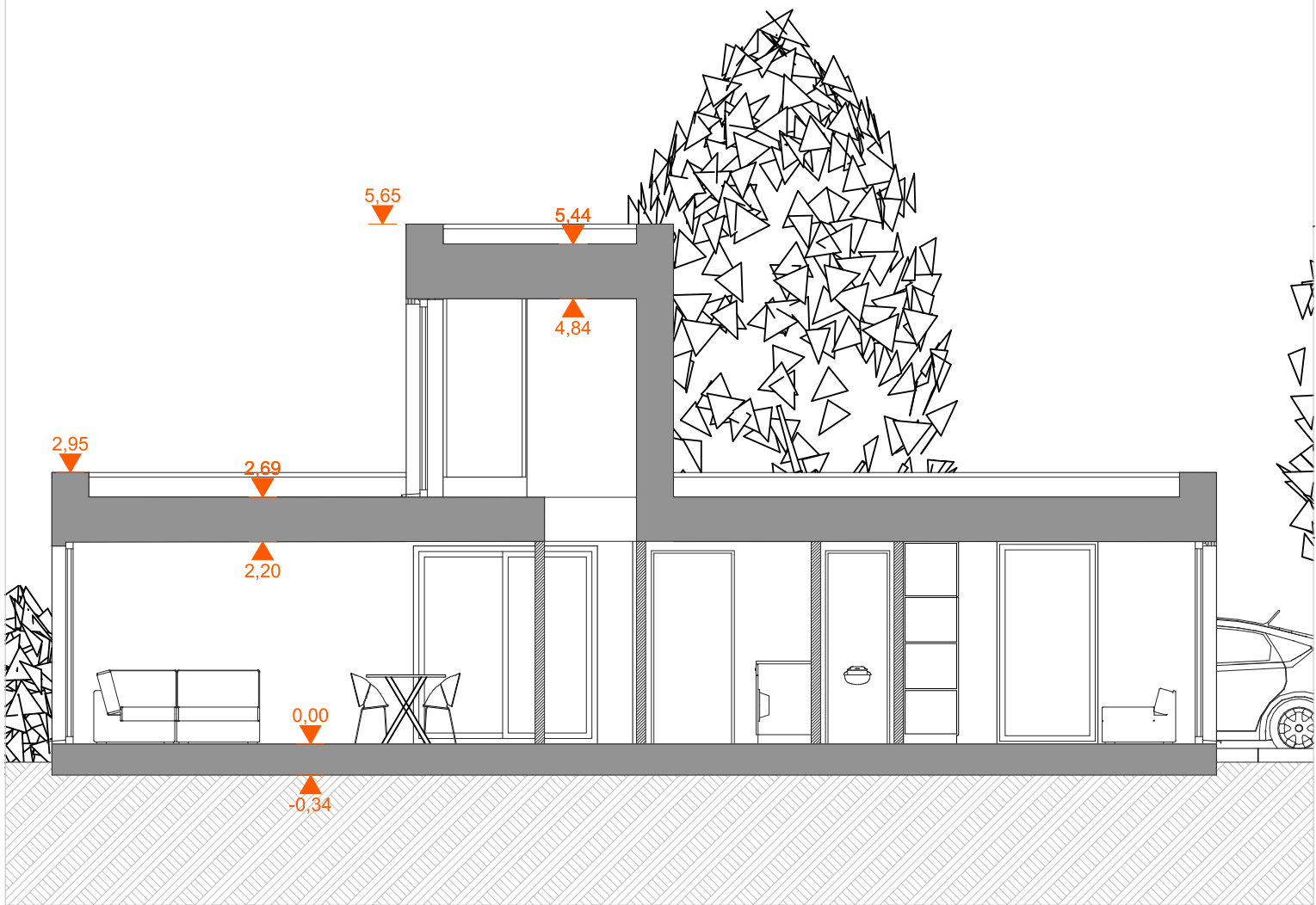
Coupe CC
