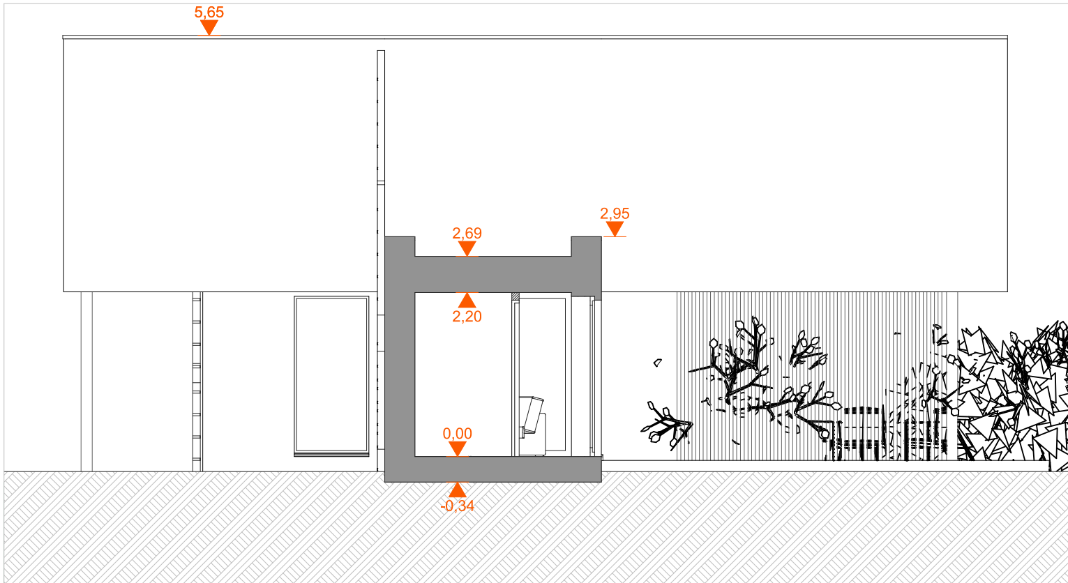
Coupe AA
