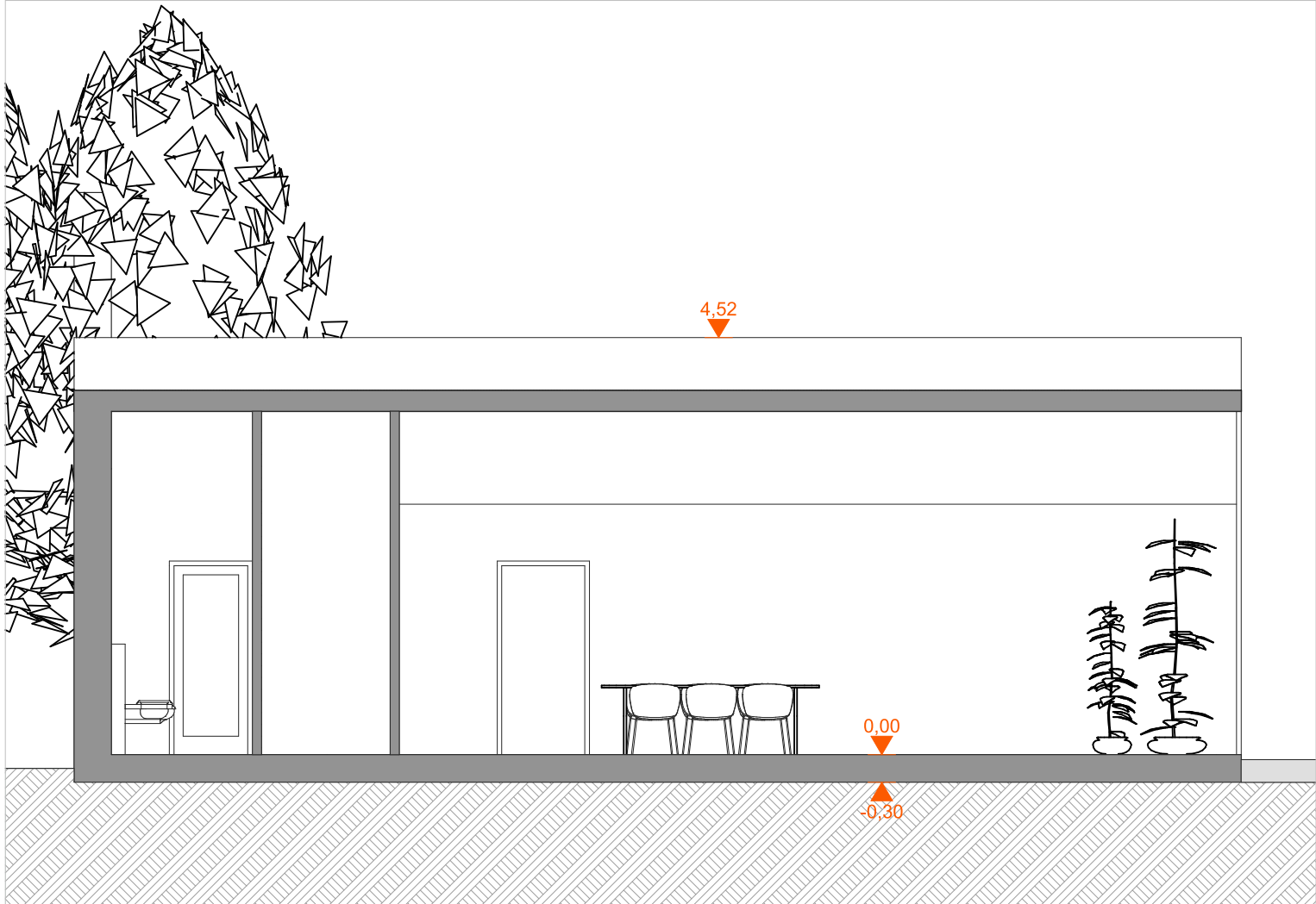
Coupe CC
