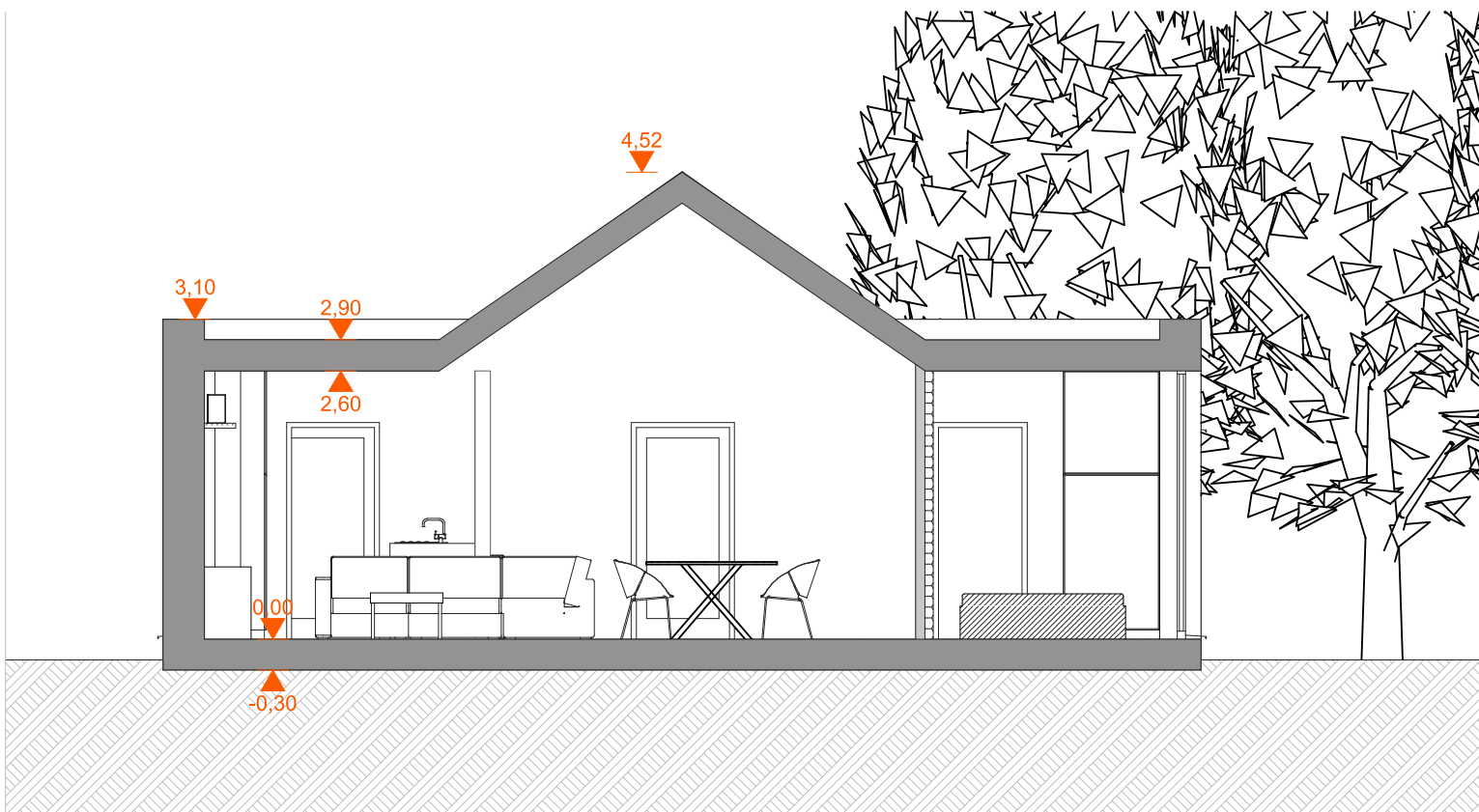
Coupe AA
