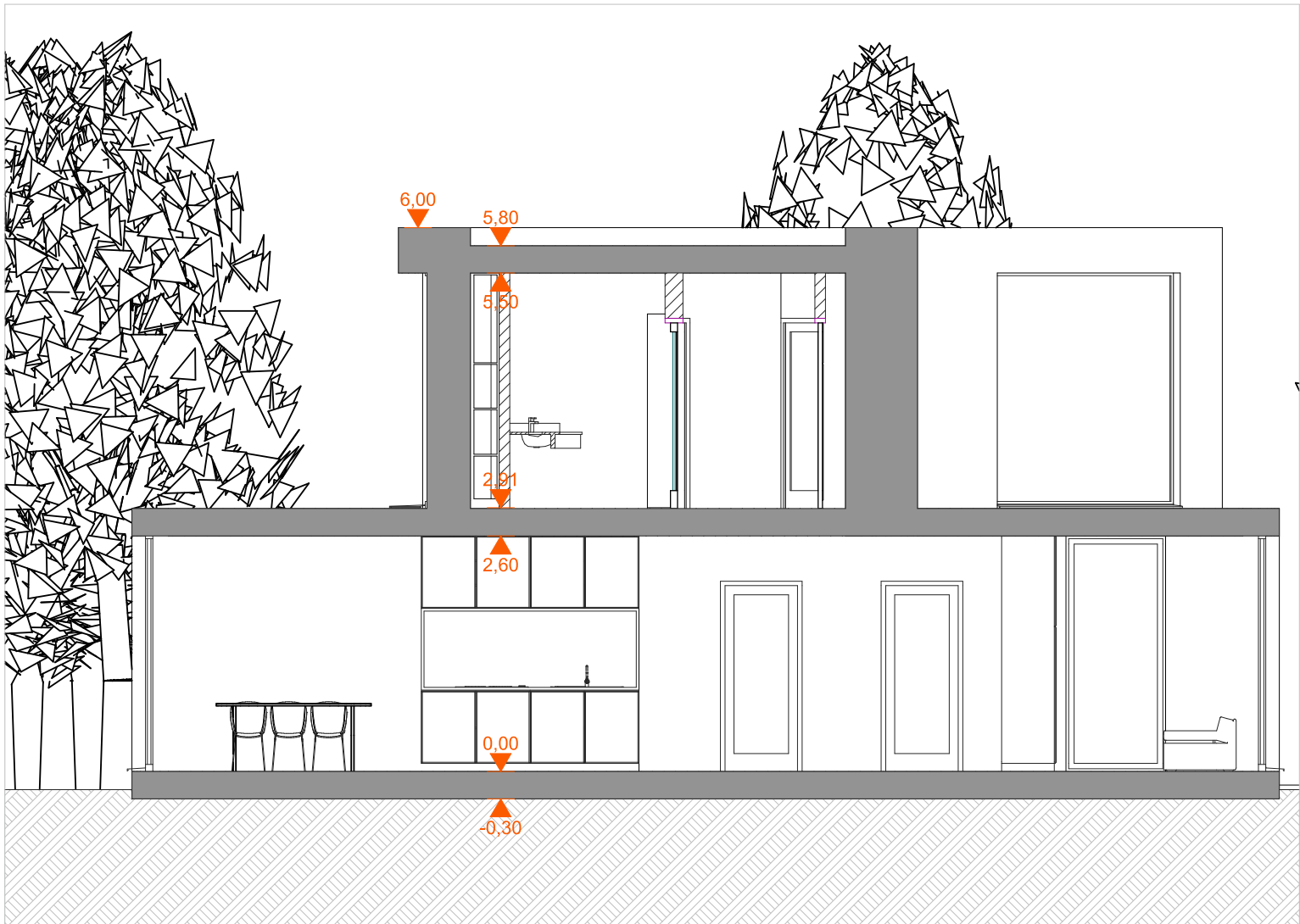
Coupe BB
